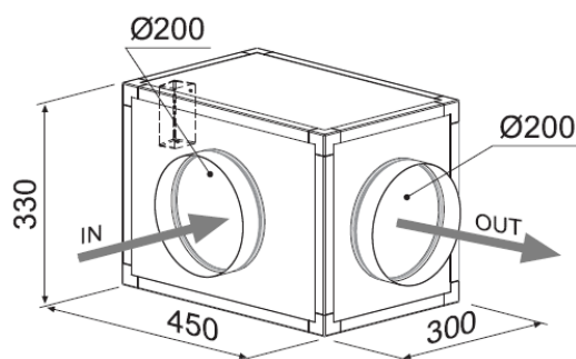
V2500 -tipo 3 (560056200017)
