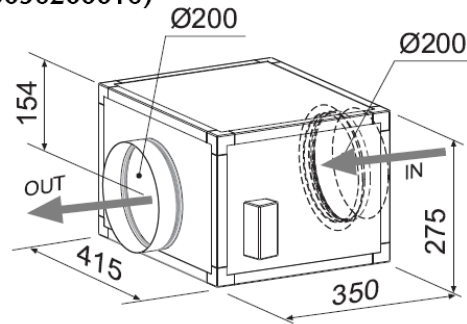
V2100 -tipo 3 (560056200009)
