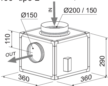
V2100 -tipo 2 (560056200009)
