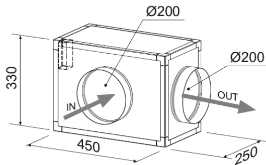
V2500 -tipo 3 (560056200017)
